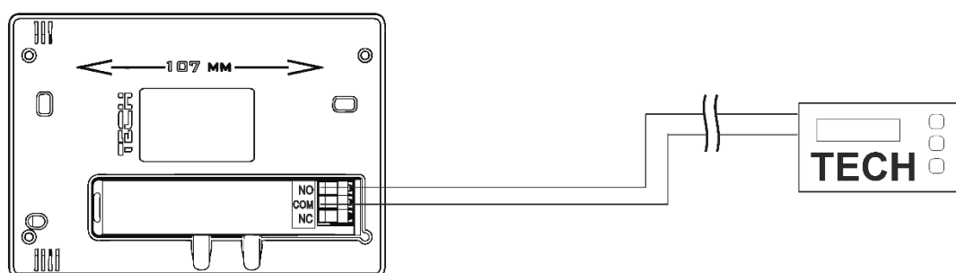
1 Schéma zapojenia regulátora CS-290 priamo s vykurovacím zariadením.
