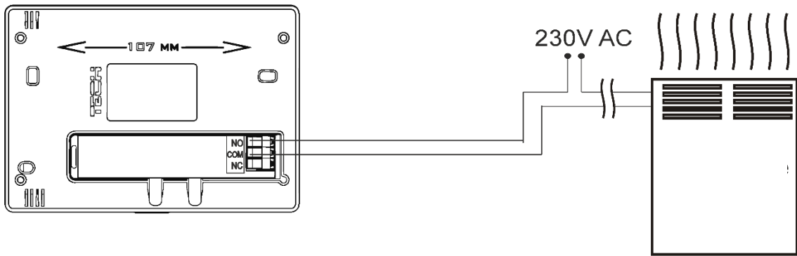
3 Schéma zapojenia regulátora CS-290 s vykurovacím zariadením so zaťažením do 1A.
