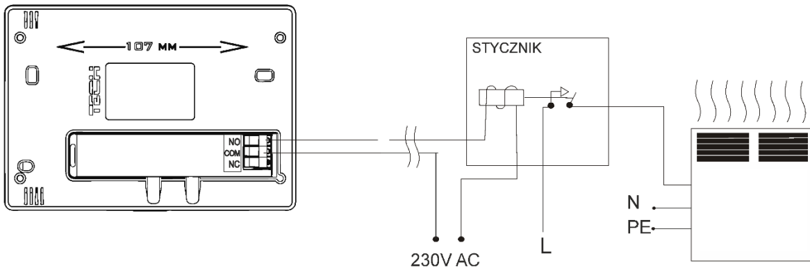
4 Schéma zapojenia regulátora CS-290 s vykurovacím zariadením so zaťažením nad 1A.
