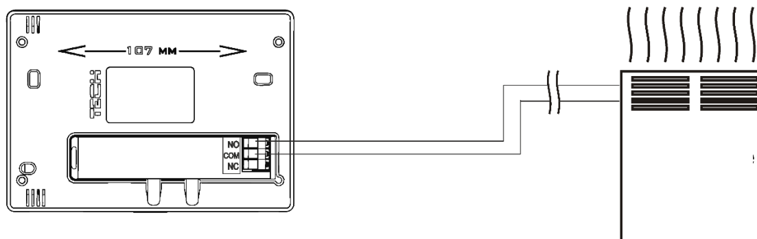
1 Schéma zapojenia regulátora CS-290 priamo s vykurovacím zariadením.
