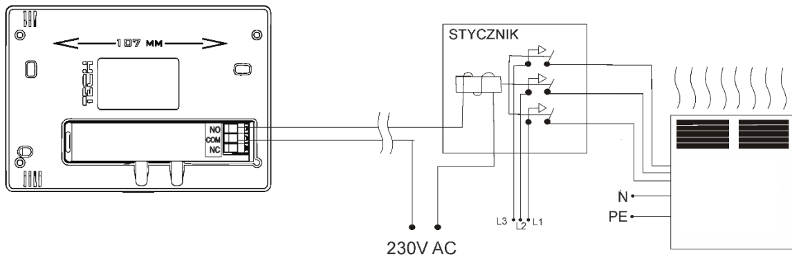
5 Schéma zapojenia regulátora CS-290 s trojfázovým vykurovacím zariadením.
