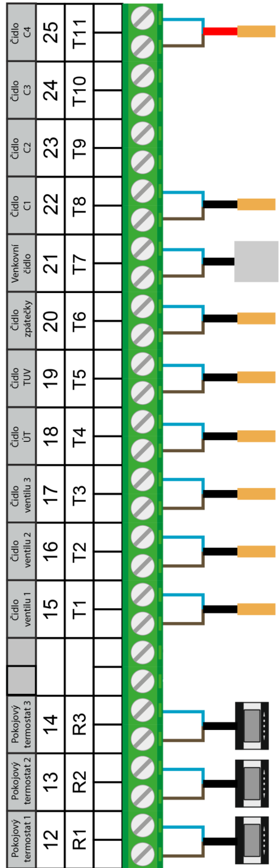
Svorkovnice regulátoru a možnosti zapojení
