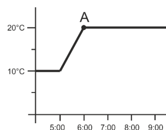
Teplota místnosti: funkce OPTIMUM START zapnutá
