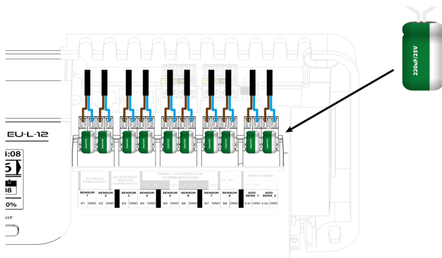
Elektrolytický kondenzátor 220 \mu F / 25 V (nízkoimpedanční)
