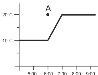
Teplota místnosti: funkce OPTIMUM START vypnutá
