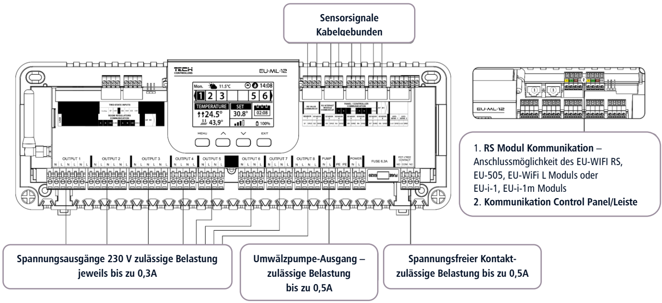
Abbildung zur Veranschaulichung des Anschlusses und der Kommunikation mit anderen Geräten in der Anlage:
