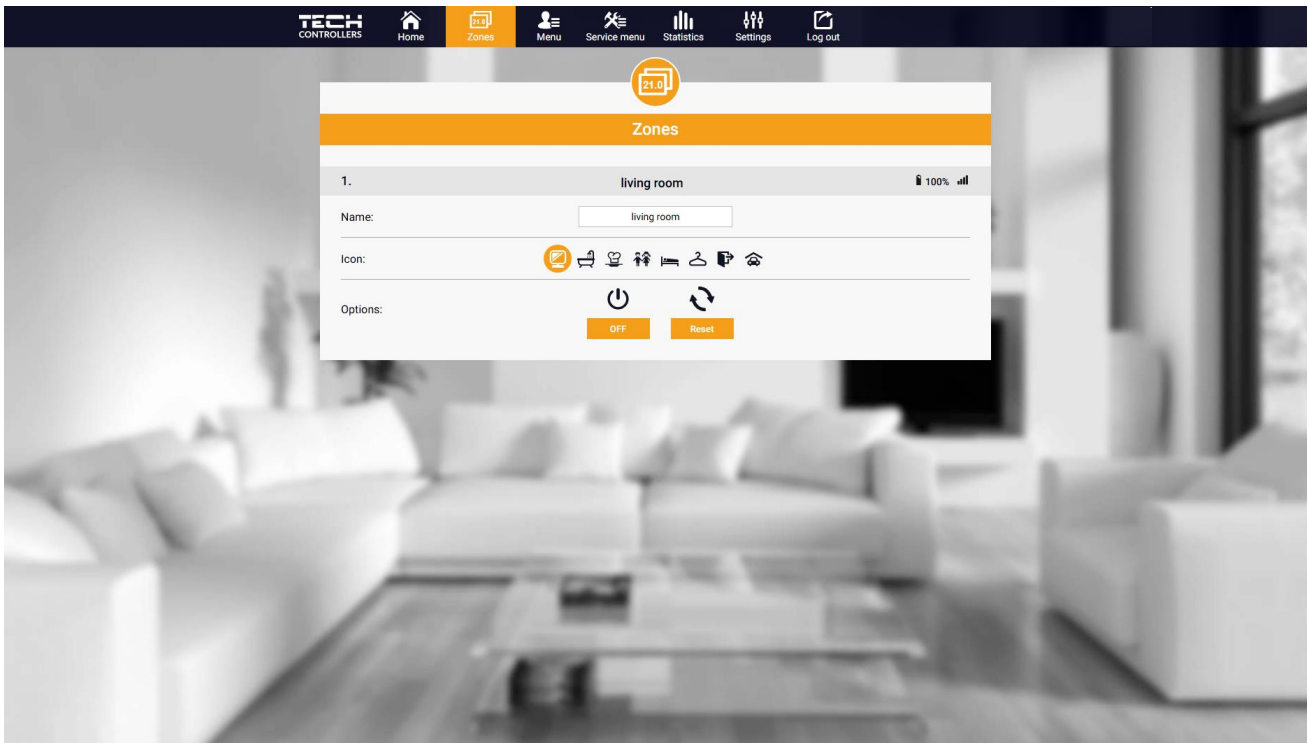
Zones tab
