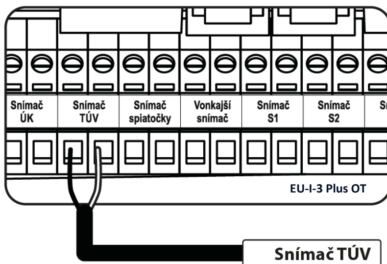
Zapojenie snímača TÚV
