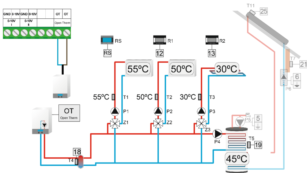
Príklad inštalácie obsluhovanej kotlom s pomocou protokolu OpenTherm
