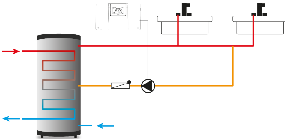
Приклад з'єднання і керування роботою циркуляційного насоса
