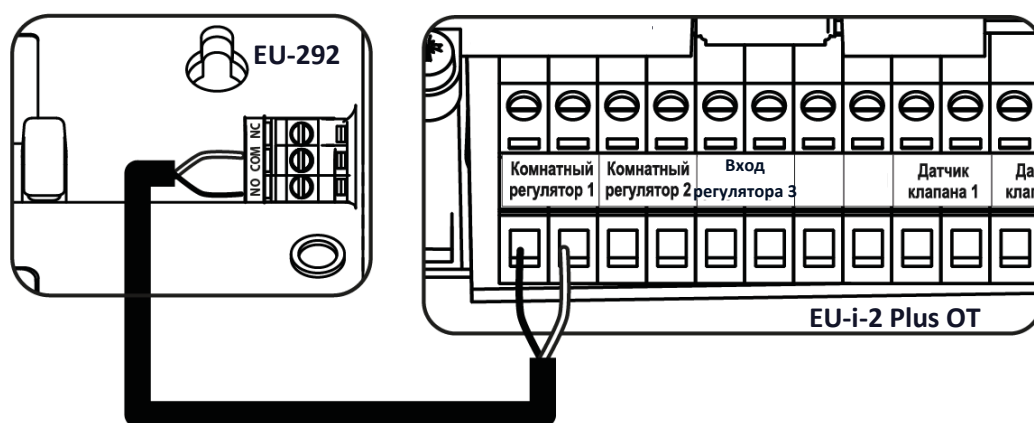
Приклад підключення дворіжнимого регулятора
