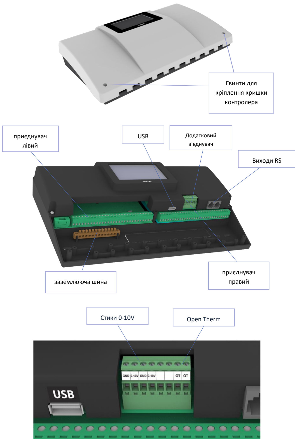
З'єднувач стиків з напругою 0 -10 V
