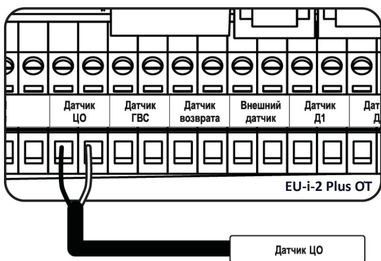
Підключення датчика ЦО
