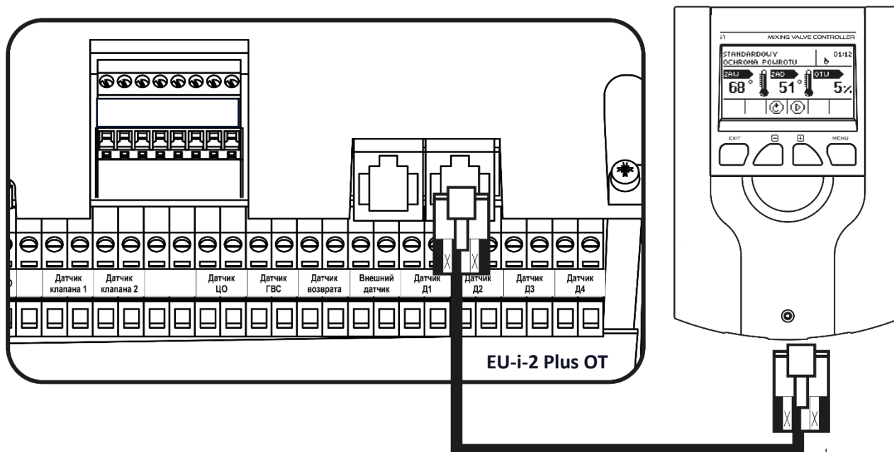
Приклад з'єднання додаткового клапана з головним контролером EU-i-2 Plus OT
