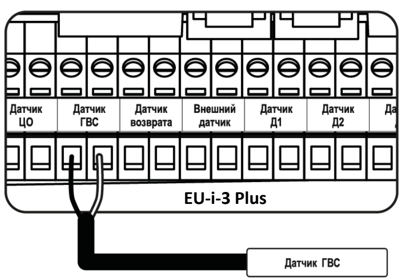
Підключення датчика ГВП
